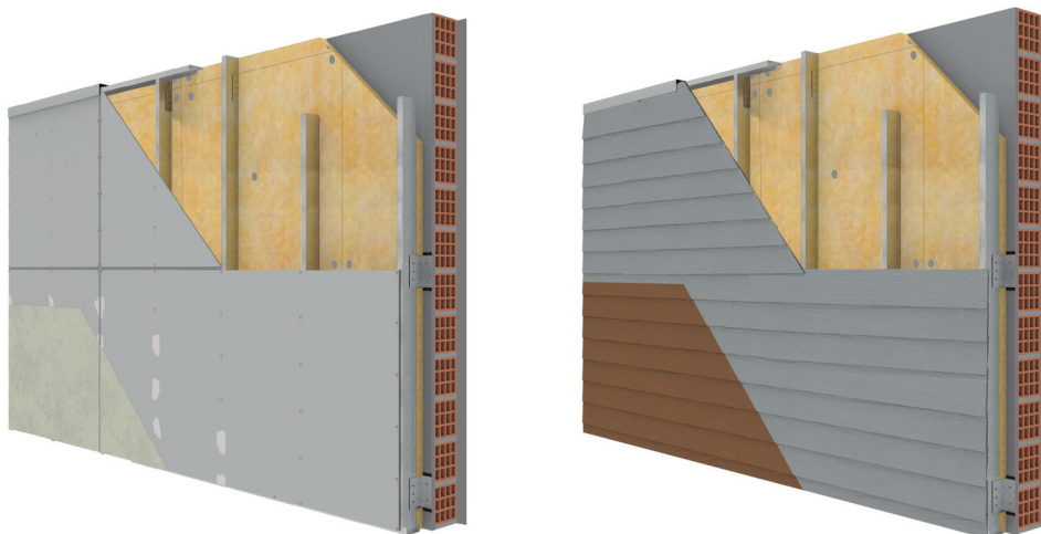
1. Placa cementicia en retrofit. 2. Siding en retrofit
