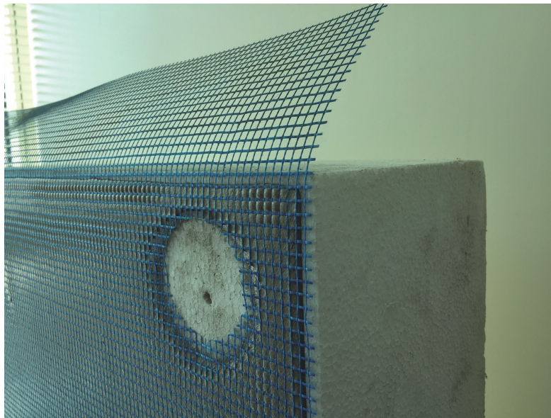
Placa termoaislante Poliestireno Expandido revestida prefabricada para EIFS
