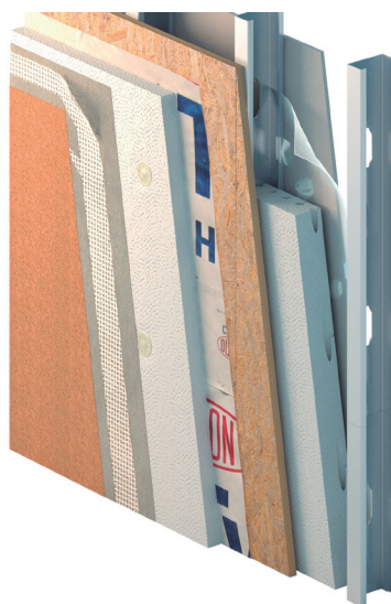
Aplicación en Sistemas en seco
