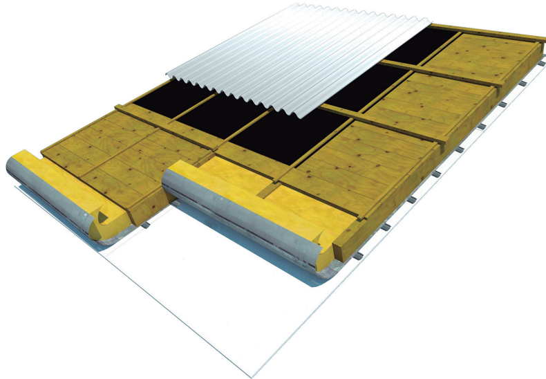
Cielorraso de Lana de vidrio paralelo a la pendiente
