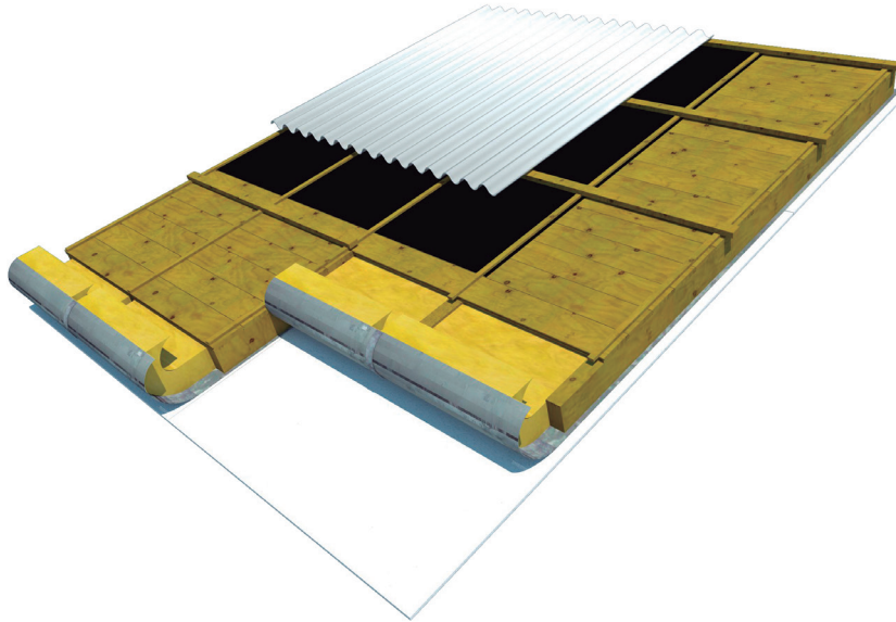
Renovación de techo de cubierta de chapa
