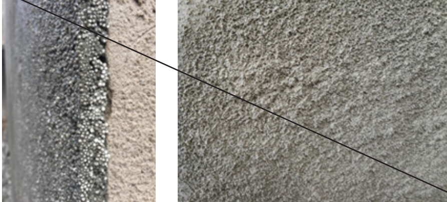
Revoque premezclado termoaislante con perlas de Poliestireno Expandido aditivadas y capacidad hidrófuga
