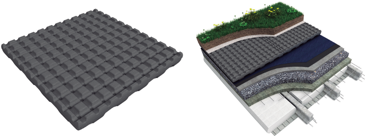
Placa termo-drenante de Poliestireno Expandido grafitada. Aplicación en techos invertidos
