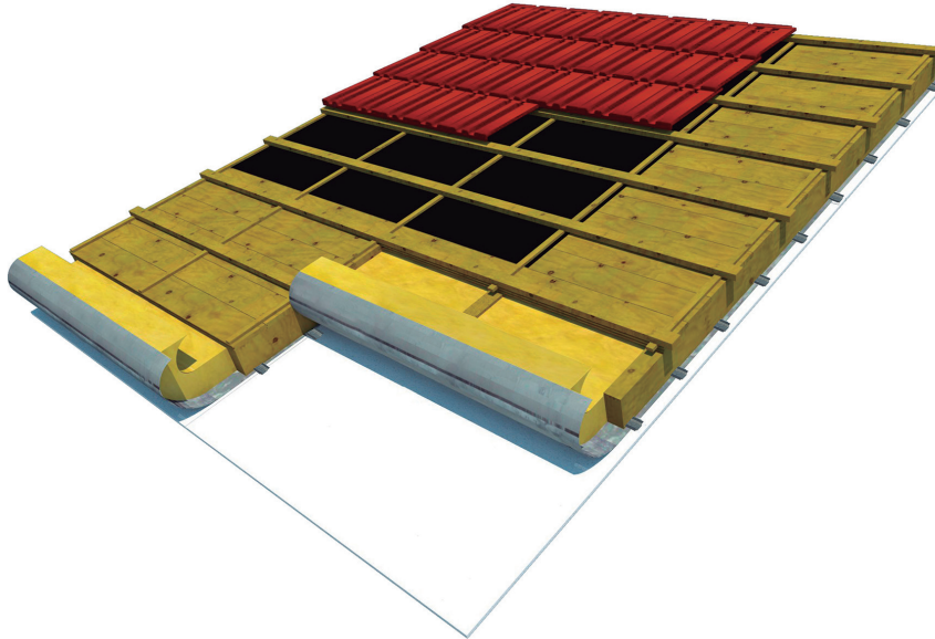
Cielorraso de Lana de vidrio paralelo a la pendiente
