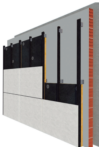
Aislamiento térmico por el exterior
