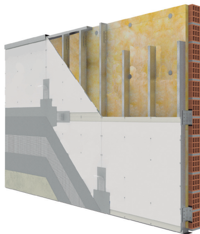
Placa de roca de yeso exteriores
