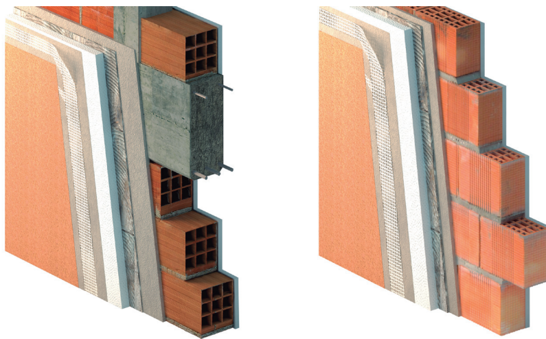
Aplicación en Sistemas húmedos
